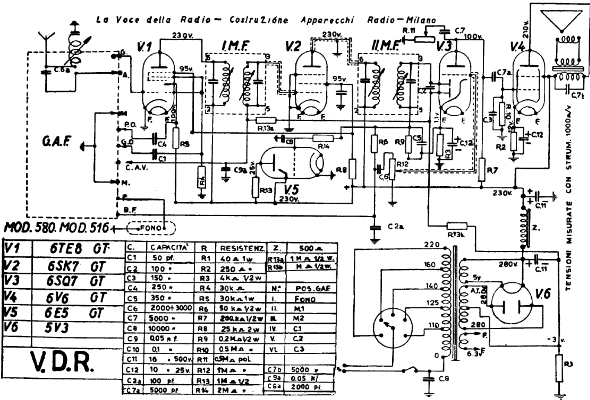
VOCE DELLA RADIO - Modd. 580, 516, 593. Onde medie I da 185 a 340 m, onde medie II da 320 a 580 m, OC1 da 16 a 25 m, OC2 da 24 a 38 m, OC3 da 35 a 55 m. Media frequenza 410 kc/s. (Il mod. 593 è provvisto di alimentatore separato). Potenza d'uscita 3,5 watt.
